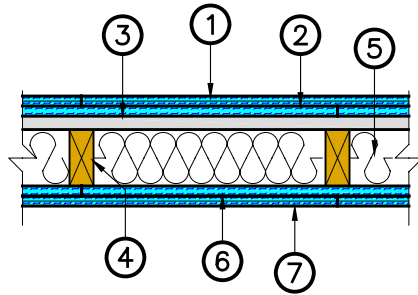
TEST# 0607 HORIZONTAL WALL SECTION SCALE: 1"=1'-0"
